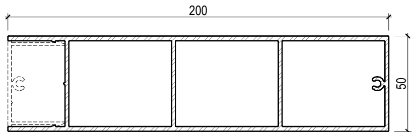
UWB20050 - ULTRAWOOD 200 x 50 Batten
