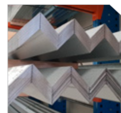
SZA/SGA**** Angles
